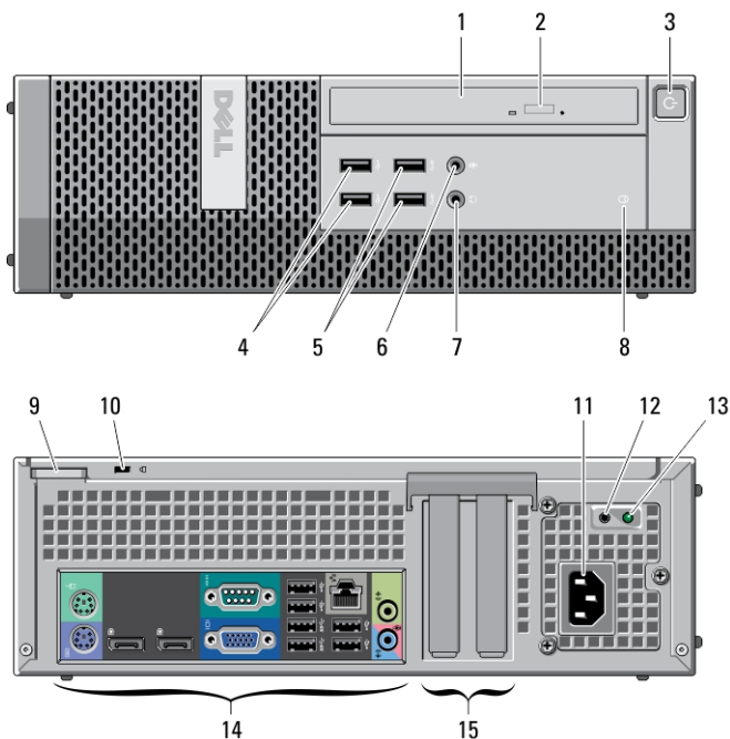
图 3: 小型计算机的背面板视图
