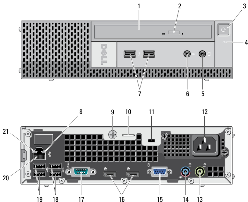
图 5: 超小型计算机的正面视图和背面视图
