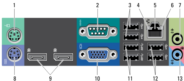
图 4: 小型计算机的背面板视图
